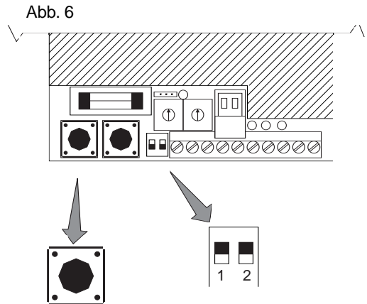
PROGRAMMIERTASTE
