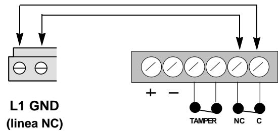
□ Fig. 9.1. Collegamento di un rivelatore (IR100), alla linea L1.
