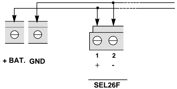
□ Fig. 2.1. Collegamenti per l'alimentazione di dispositivi tipo SEL26F (sirene autoalimentate)
