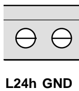
□ Fig. 8. Linea L24h (antisabotaggio) NC, istantanea.
